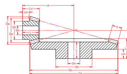
1:4 Mat. C45
