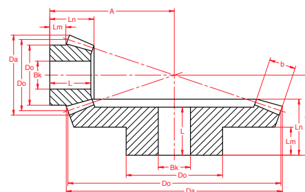
1:3 Mat. C45
