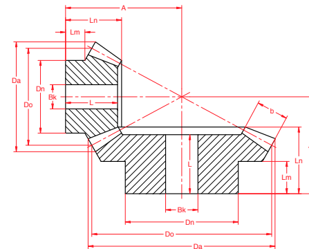
1:2 Mat. C45
