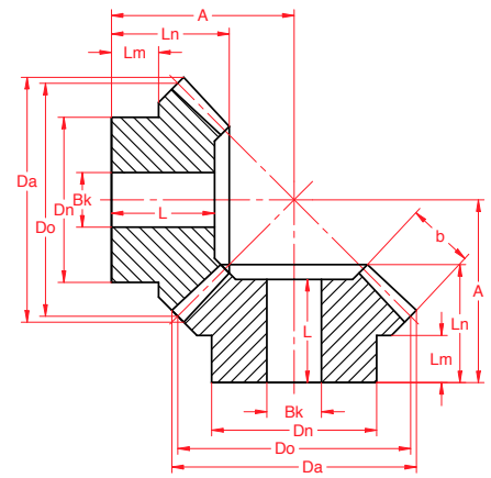
1:1 Mat. C45
